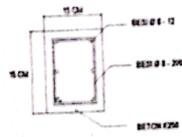
DETAIL KOLOM 15X15
