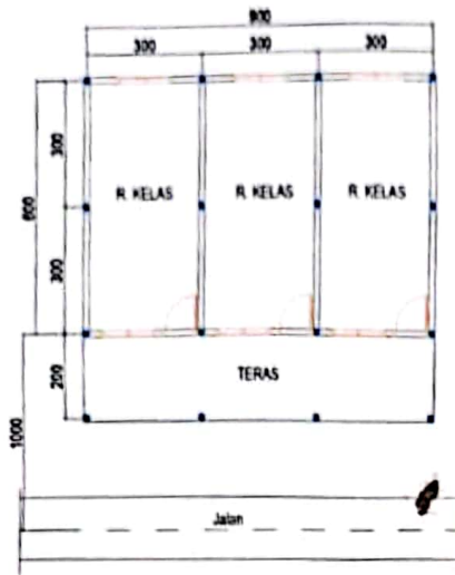
DENAH BANGUNAN
