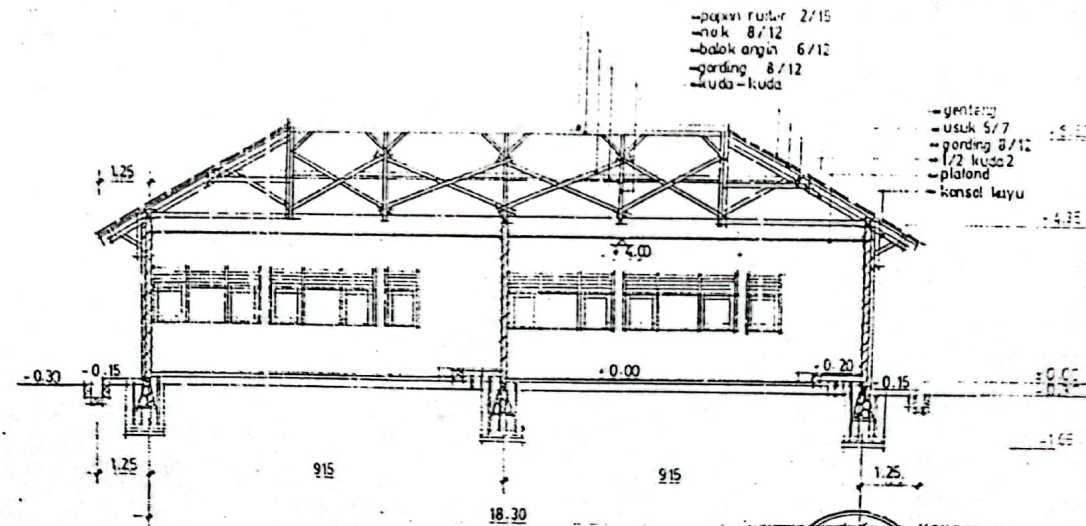
# POTONGAN SKALA 1 : 100
