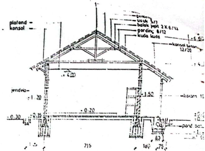
# POTONGAN 01 SKALA 1 : 100
