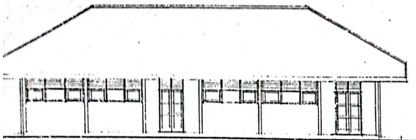
# TAMPAK DEPAN SKALA 1 : 100
